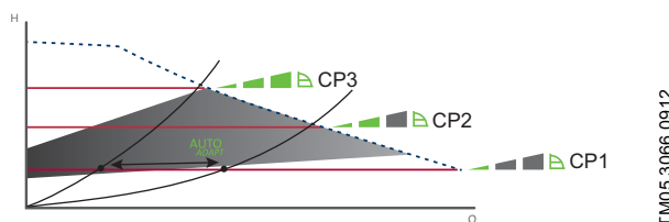
Abb. 19 Die drei Konstantdruck-Kennlinien/-Einstellungen
