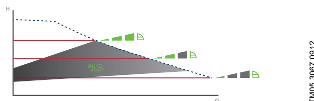
Abb. 18 Auswählen der Pumpeneinstellung in Abhängigkeit der vorliegenden Anlage
