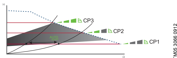
Abb. 17 Die drei Konstantdruck-Kennlinien/-Einstellungen
