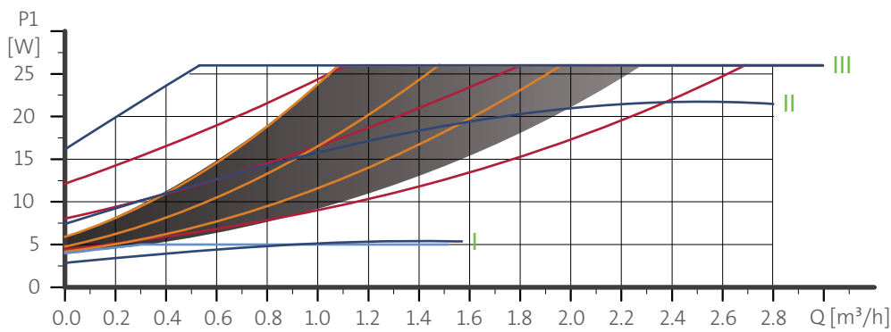
Abb. 31 ALPHA2 XX-50
