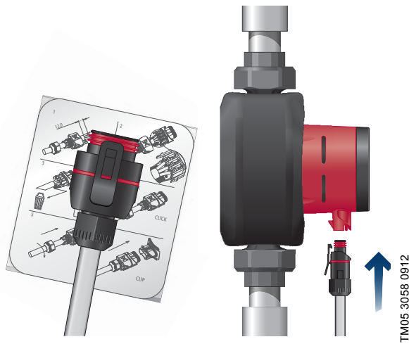
Abb. 9 Elektrischer Anschluss
