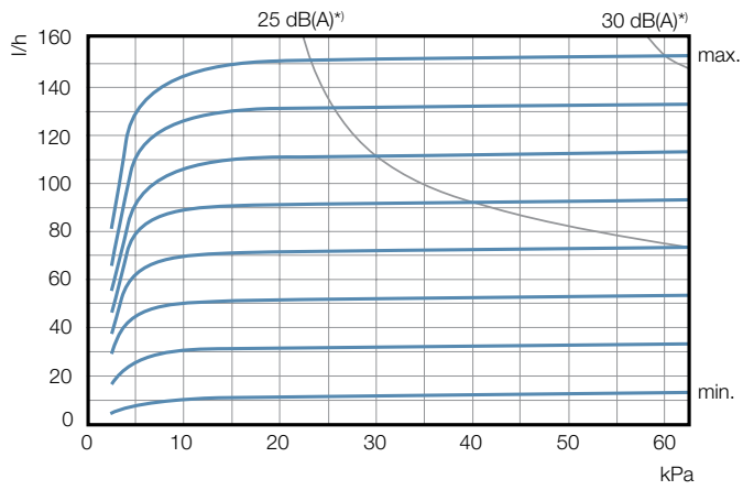
Geringste Durchflusstoleranzen
