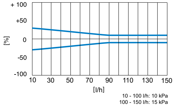
Geringste Durchflusstoleranzen
