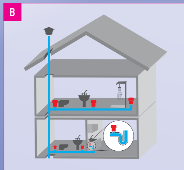
Prinzip der Belüftungsventil in Pflanzen Sanitärinstallation mit Abgasanlagen
