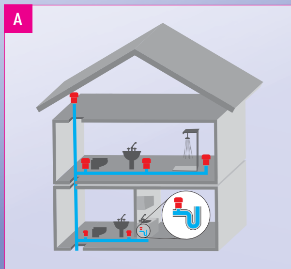
Prinzip der Belüftungsventil in Pflanzen Sanitärinstallation ohne Abgasanlagen
